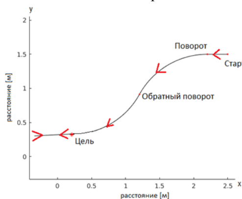
Рис. 8. Траектория движения модели робомобиля Uniор
