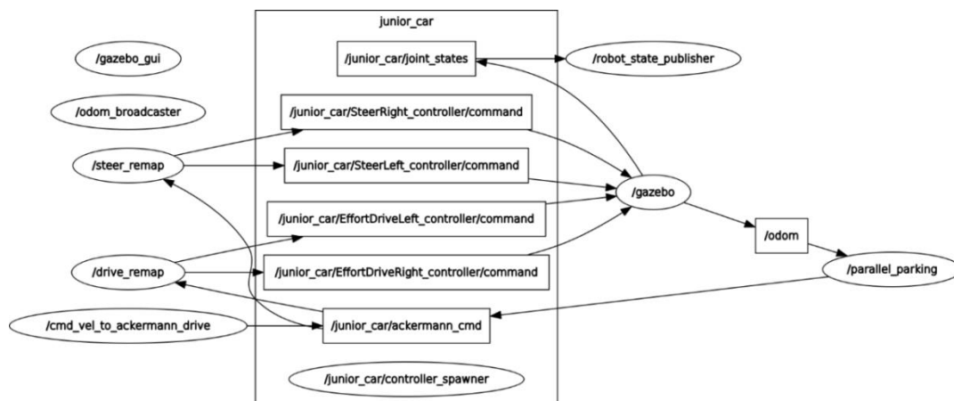
Рис. 4. Архитектура ROS модели робомобиля Unior (из Робототехнической Операционной системы (ROS))
